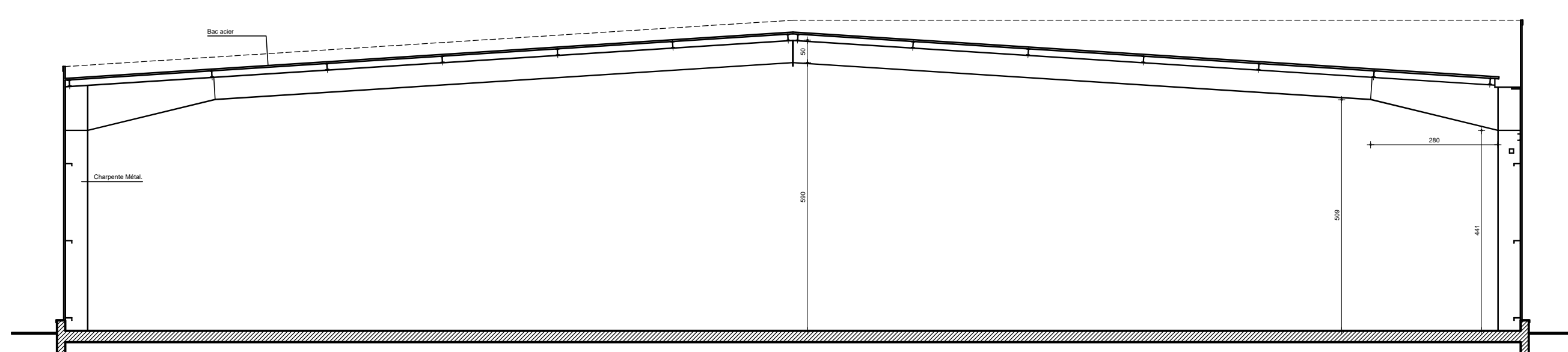
BATIMENT C COUPE A.A.
